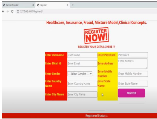
Fig.2. Register page.
