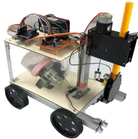
Fig.1. Hardware kit.
